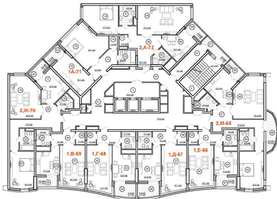
План поверху, М 1:200
