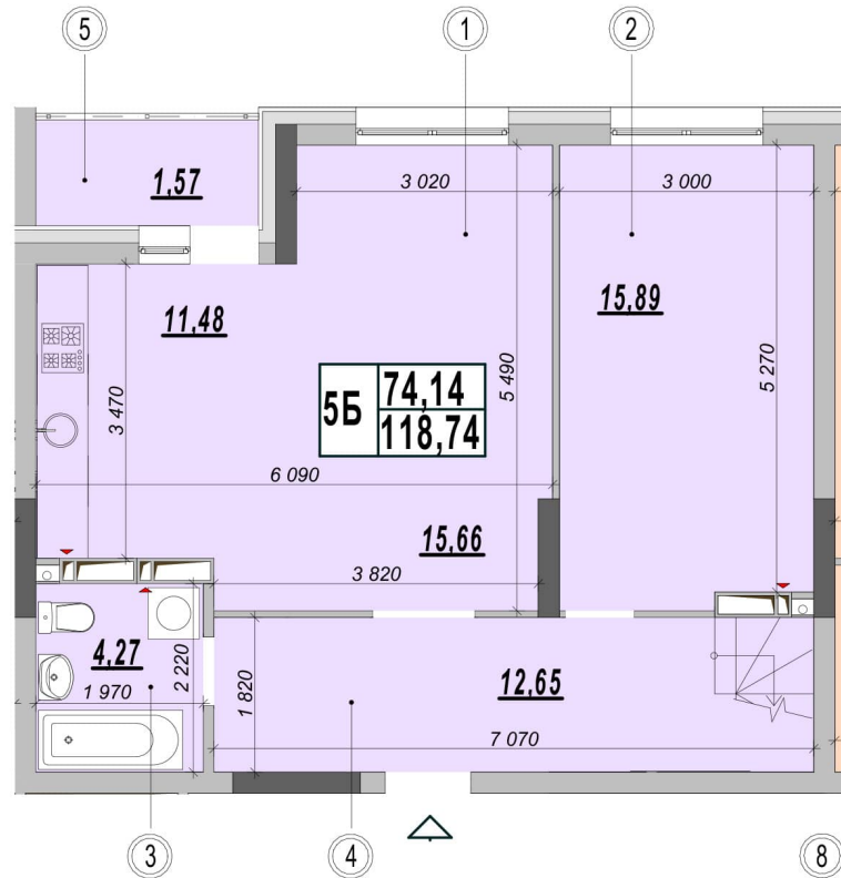
План секції 1.2
